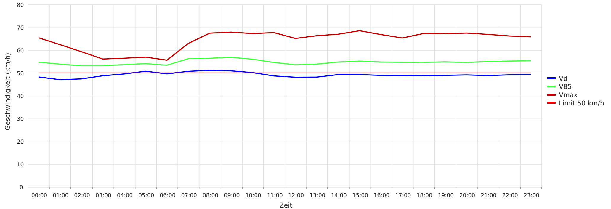
2025_06_04-2025_07_01 Bothmer Richtung Schwarmstedt Vd, V85, Vmax vs. Uhrzeit
