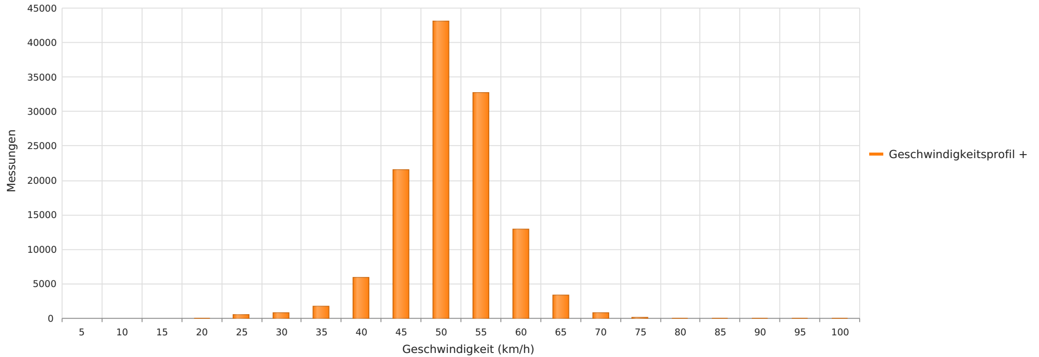
2025_06_04-2025_07_01 Bothmer Richtung Schwarmstedt Anzahl der Messwerte vs. Geschwindigkeit
