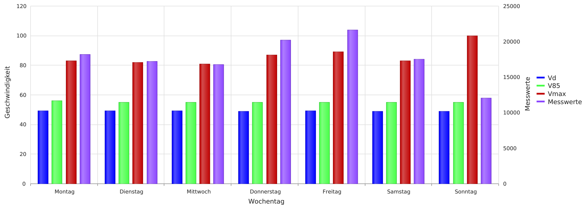
2025_06_04-2025_07_01 Bothmer Richtung Schwarmstedt Vd, V85, Vmax, Anzahl der Messwerte vs. Wochentag
