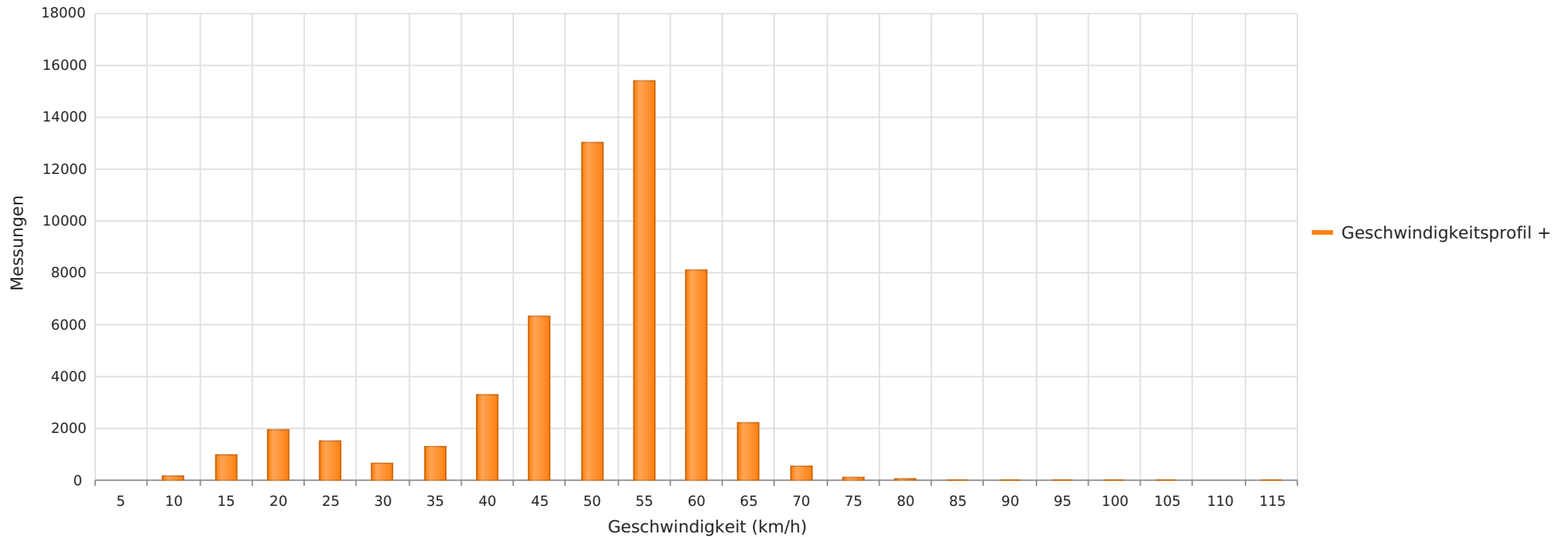
2025_06_04-2025_07_01 Bothmer Richtung Gilten Anzahl der Messwerte vs. Geschwindigkeit
