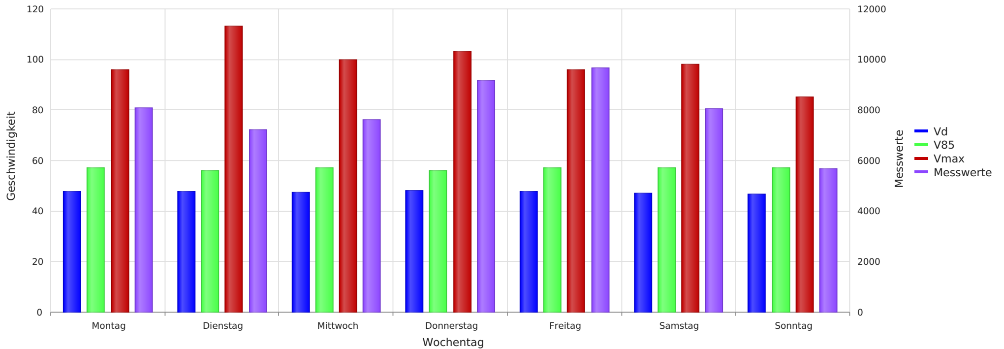
2025_06_04-2025_07_01 Bothmer Richtung Gilten Vd, V85, Vmax, Anzahl der Messwerte vs. Wochentag
