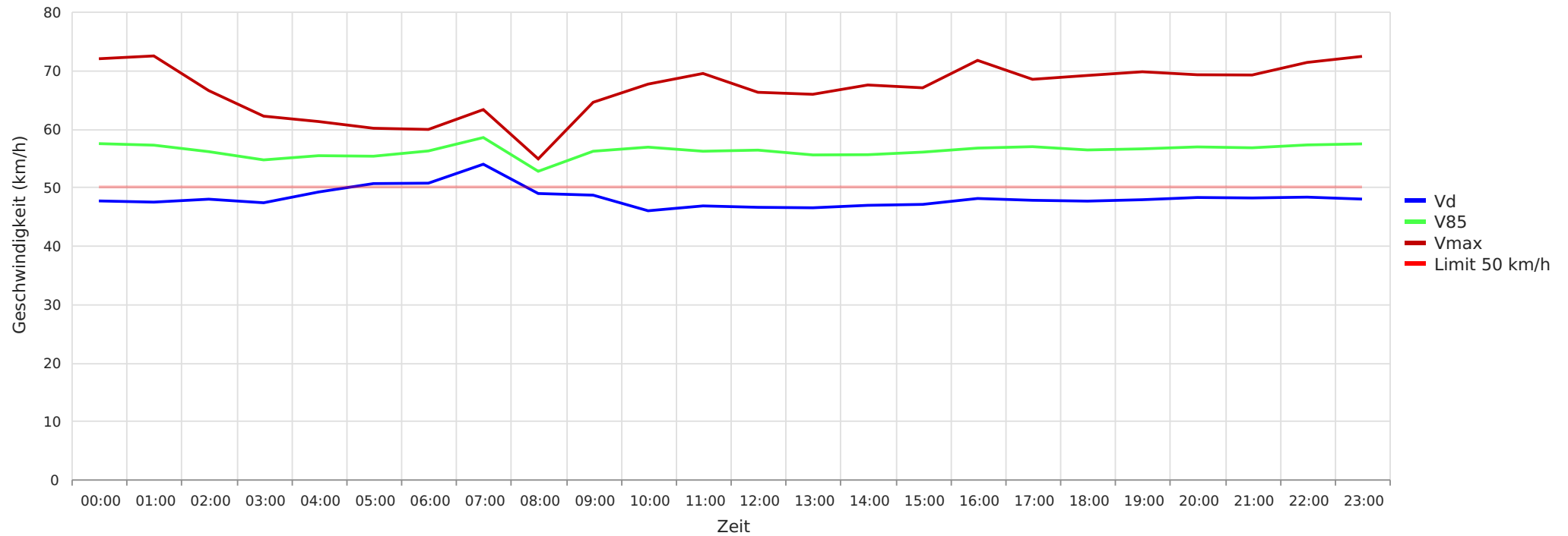
2025_06_04-2025_07_01 Bothmer Richtung Gilten Vd, V85, Vmax vs. Uhrzeit
