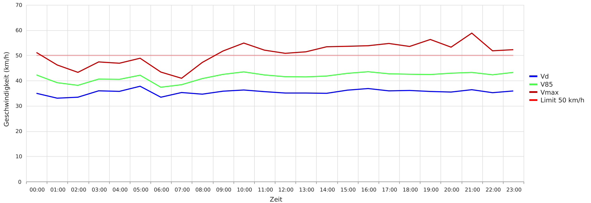
2025_06_03-2025_06_19 Buchholz_Westerholzstr. Richtung B214 Vd, V85, Vmax vs. Uhrzeit
