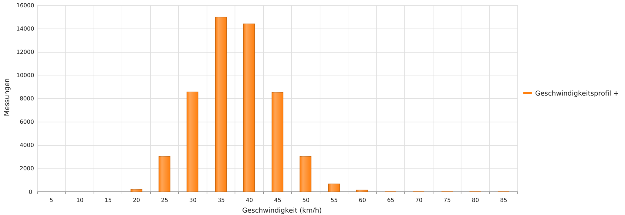
2025_06_03-2025_06_19 Buchholz_Westerholzstr. Richtung B214 Anzahl der Messwerte vs. Geschwindigkeit
