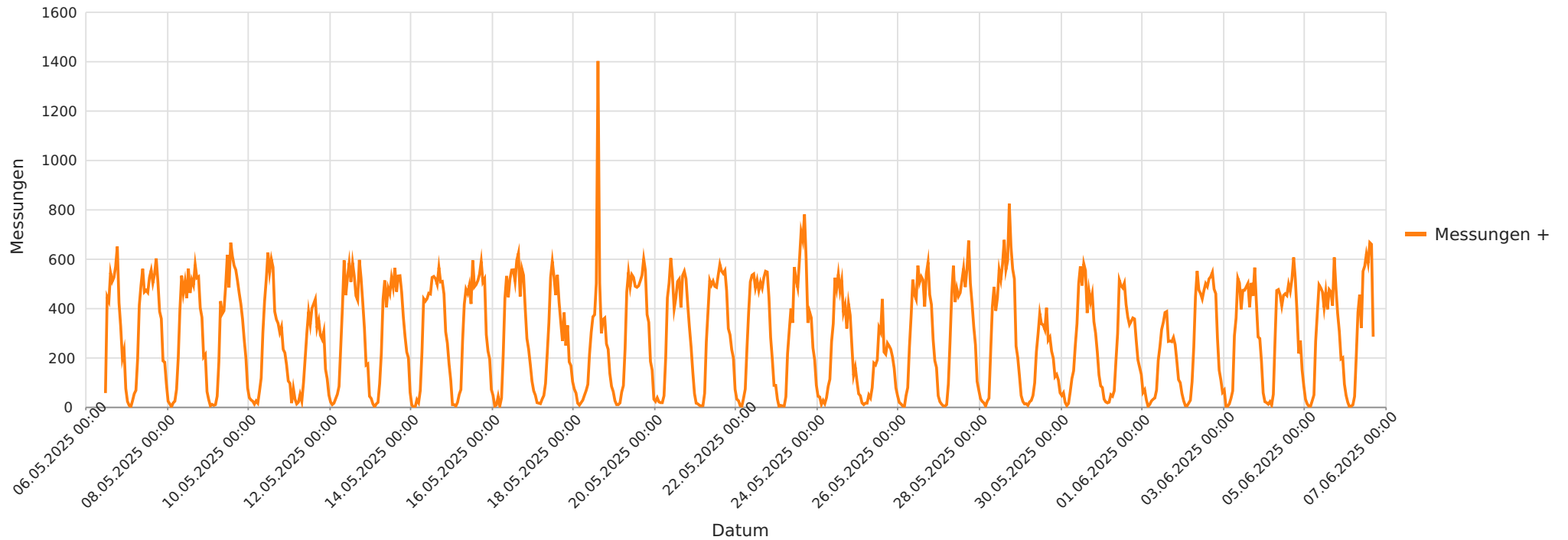
2025_05_06-2025_06_06 Essel K105 Richtung Ortskern Anzahl der Messwerte vs. Messzeitraum
