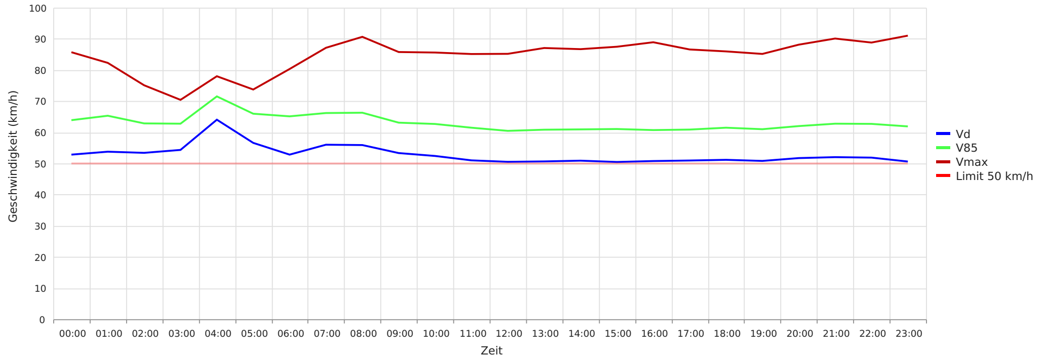
2025_05_06-2025_06_06 Essel K105 Richtung Ortskern Vd, V85, Vmax vs. Uhrzeit
