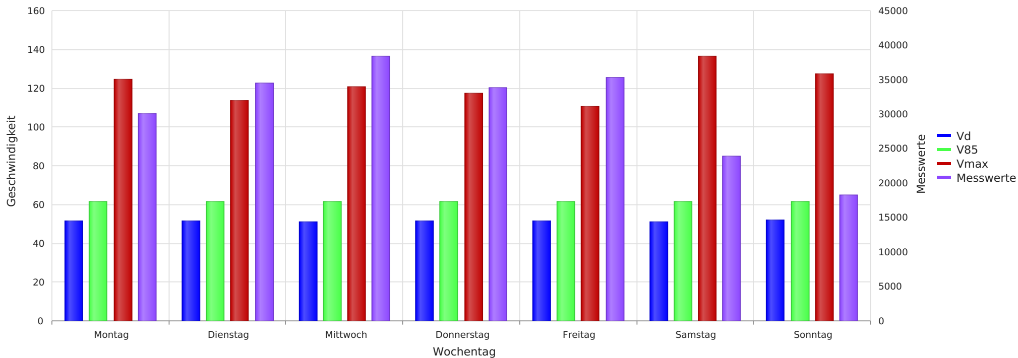
2025_05_06-2025_06_06 Essel K105 Richtung Ortskern Vd, V85, Vmax, Anzahl der Messwerte vs. Wochentag
