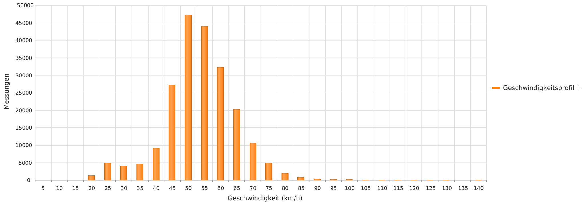
2025_05_06-2025_06_06 Essel K105 Richtung Ortskern Anzahl der Messwerte vs. Geschwindigkeit
