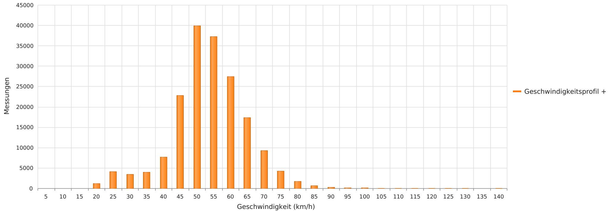
2025_05_06-2025_06_02 Essel, K105 Richtung Ortskern Anzahl der Messwerte vs. Geschwindigkeit
