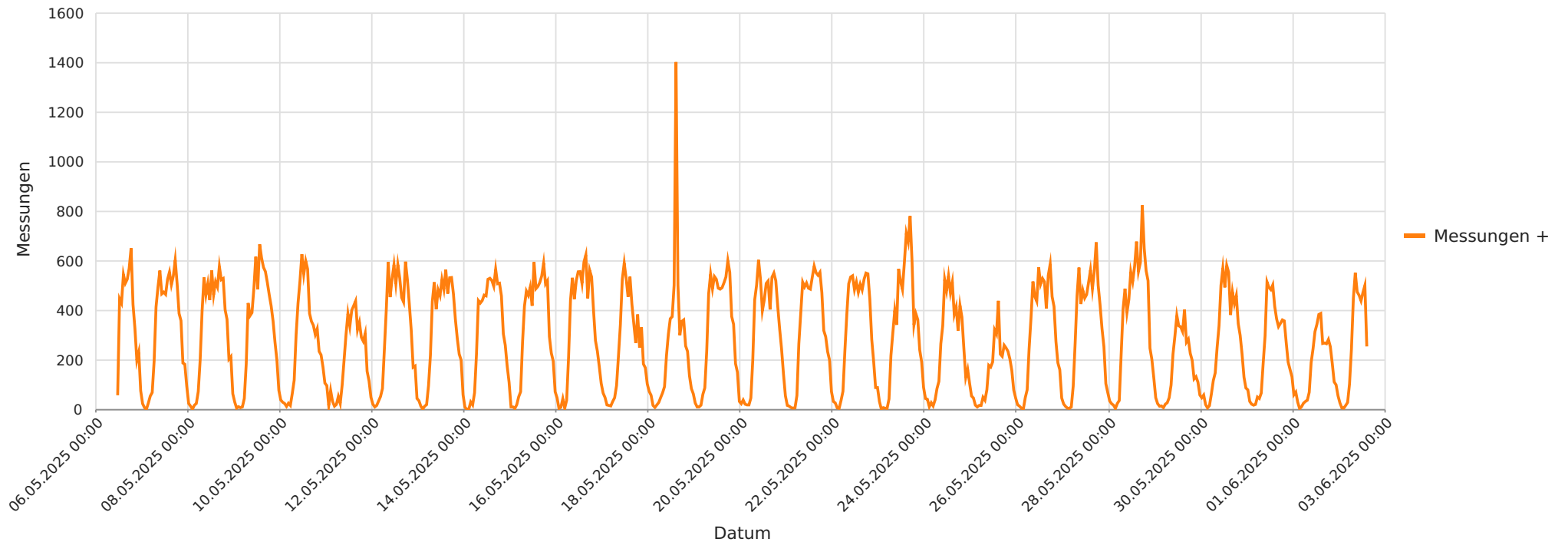
2025_05_06-2025_06_02 Essel, K105 Richtung Ortskern Anzahl der Messwerte vs. Messzeitraum
