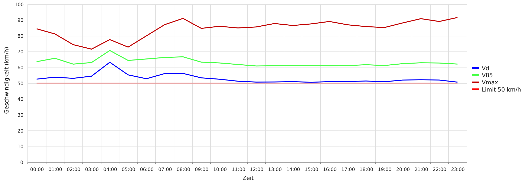
2025_05_06-2025_06_02 Essel, K105 Richtung Ortskern Vd, V85, Vmax vs. Uhrzeit
