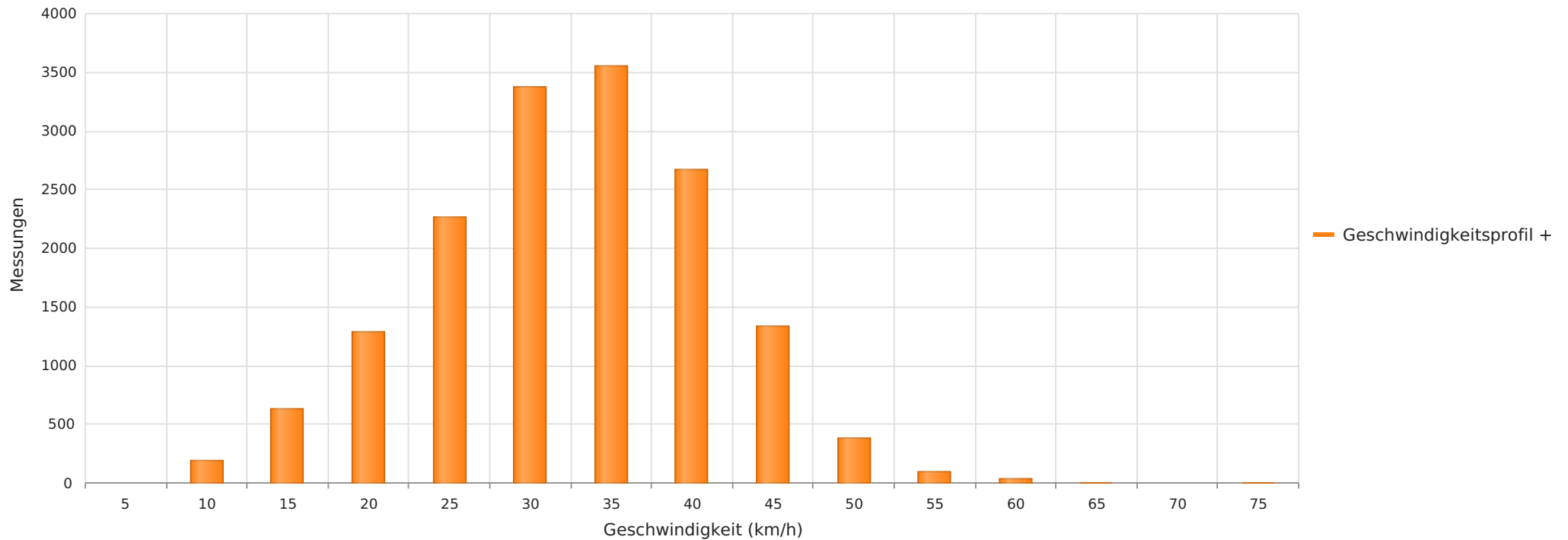
2025_04_09-2025_05_17 Marklendorf, Meierweg Richtung Jeversen Anzahl der Messwerte vs. Geschwindigkeit
