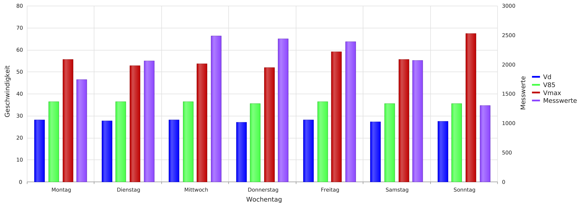
2025_04_09-2025_05_17 Marklendorf, Meierweg Richtung Jeverzen Vd, V85, Vmax, Anzahl der Messwerte vs. Wochentag
