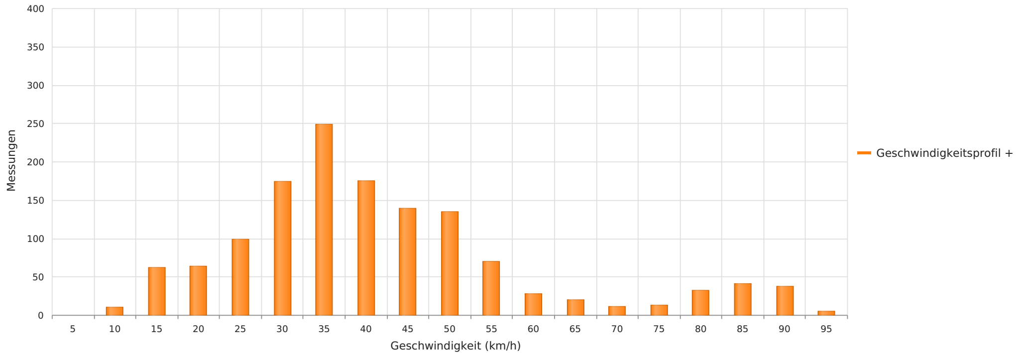
2025_03_06-2025_03_24 Grindau, Heimat zoo Richtung Buchholzer Mühlenweg Anzahl der Messwerte vs. Geschwindigkeit
