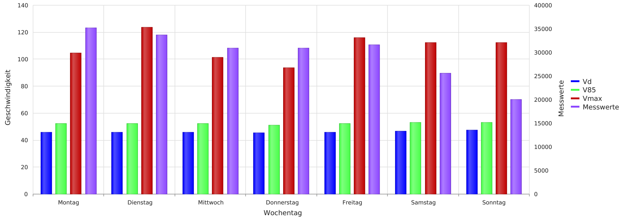
2025_03_10-2025_04_01, Buchholz B214, Richtung Celle Vd, V85, Vmax, Anzahl der Messwerte vs. Wochentag
