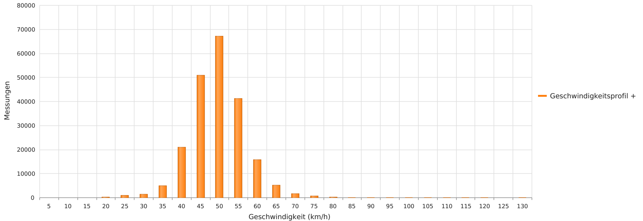
2025_03_10-2025_04_01, Buchholz B214, Richtung Celle Anzahl der Messwerte vs. Geschwindigkeit
