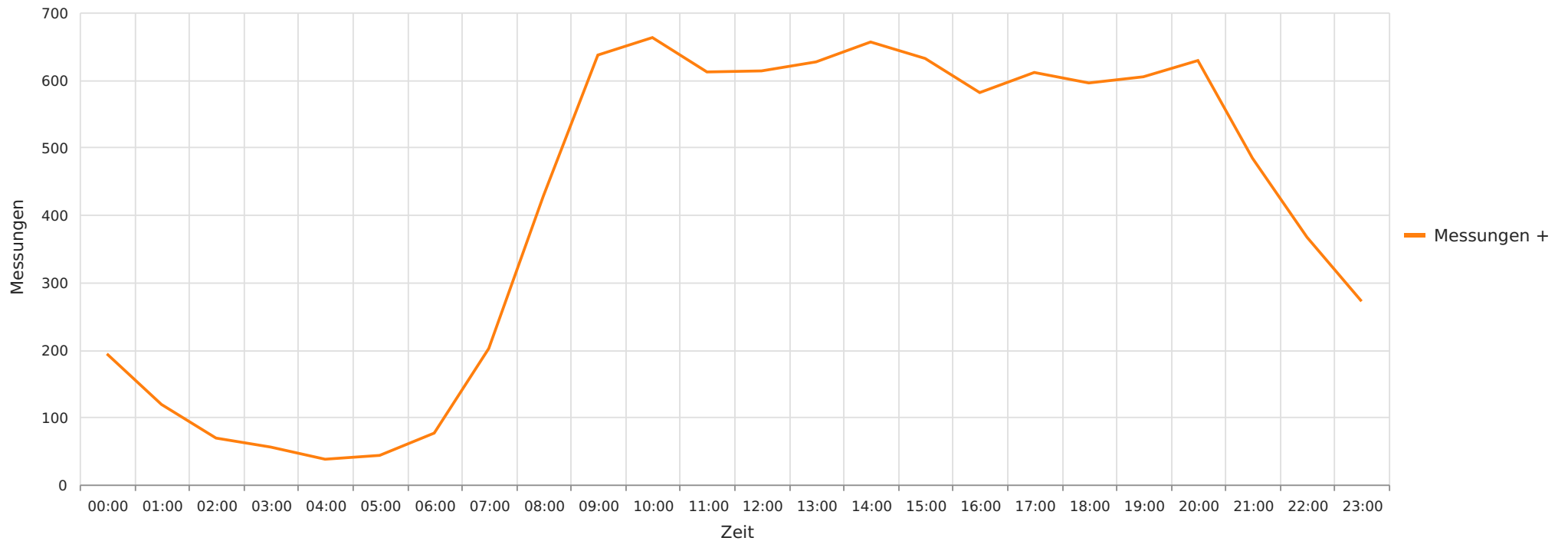
2025_03_10-2025_04_01, Buchholz B214, Richtung Celle Gemittelte Anzahl an Messwerten vs. Uhrzeit
