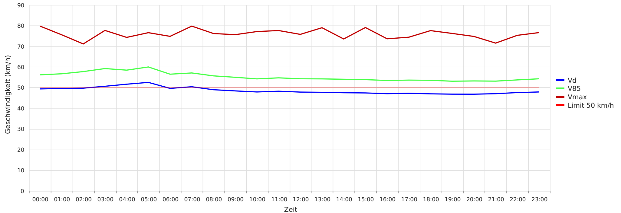
2025_03_10-2025_04_01, Buchholz B214, Richtung Celle Vd, V85, Vmax vs. Uhrzeit
