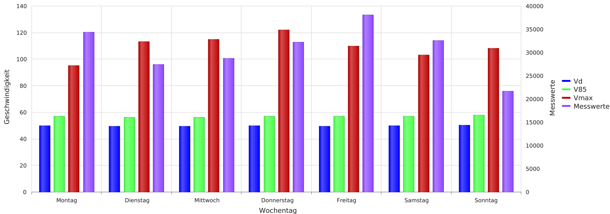
2025_03_06-2025_03_31 Grindau, L193 Richtung Ortskern Vd, V85, Vmax, Anzahl der Messwerte vs. Wochentag
