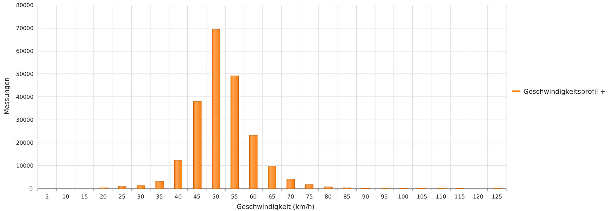
2025_03_06-2025_03_31 Grindau, L193 Richtung Ortskern Anzahl der Messwerte vs. Geschwindigkeit
