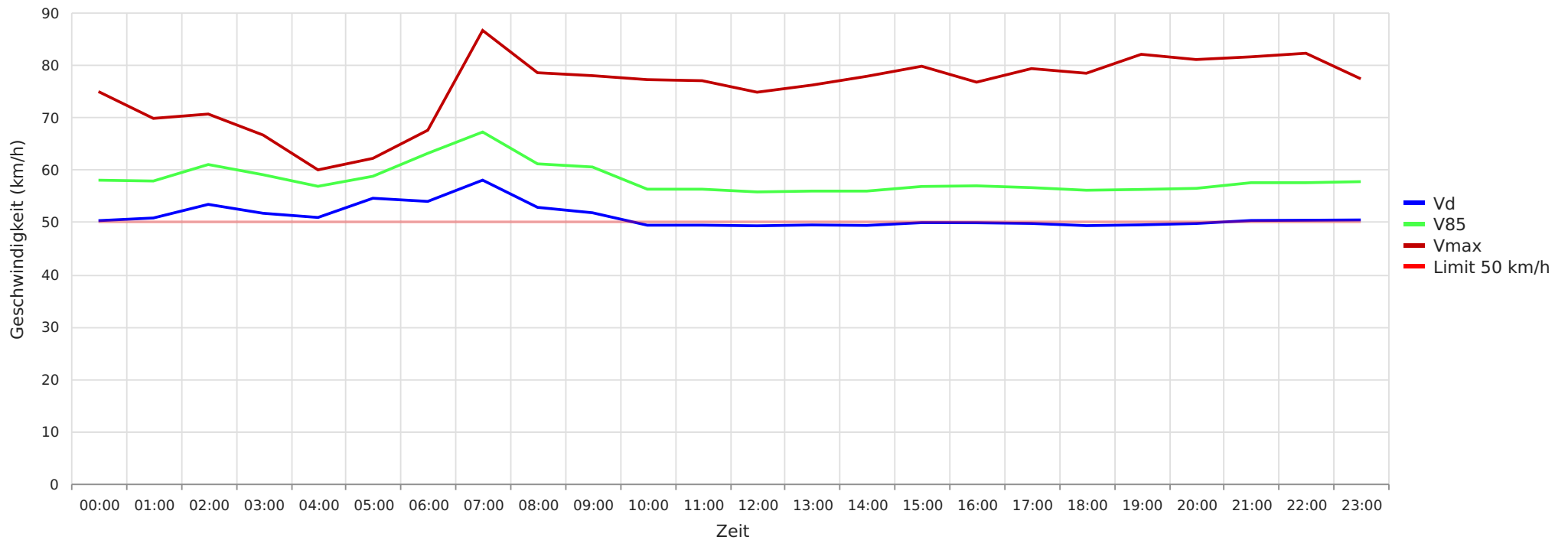
2025_03_06-2025_03_31 Grindau, L193 Richtung Ortskern Vd, V85, Vmax vs. Uhrzeit
