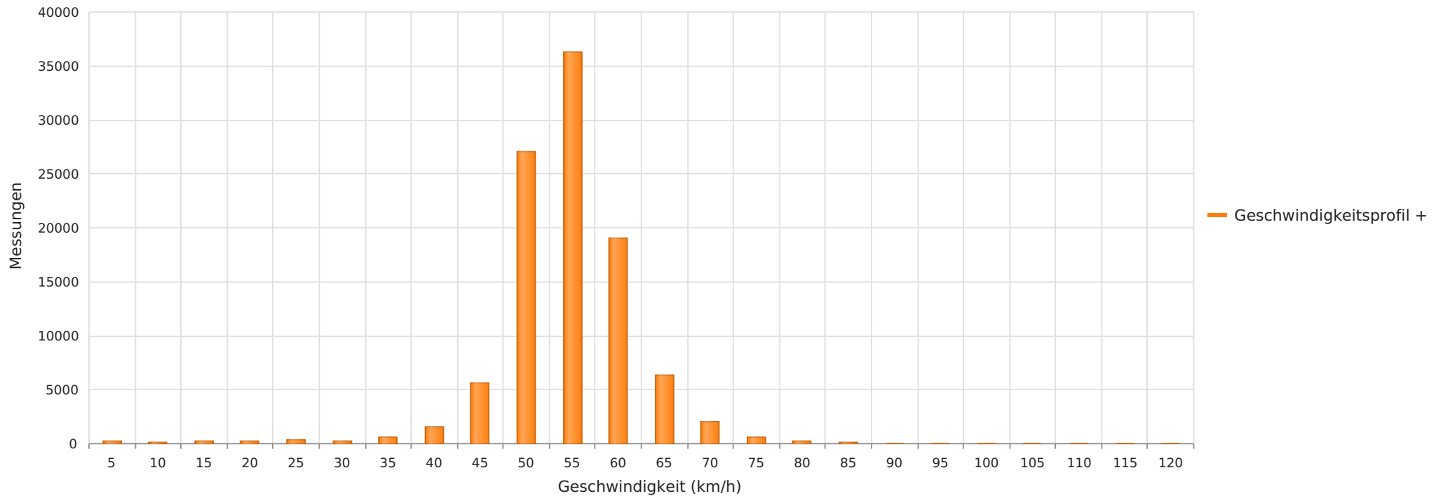
2024_12_13-2025_03_11 Norddrebber B214 Richtung Schwarmstedt Anzahl der Messwerte vs. Geschwindigkeit
