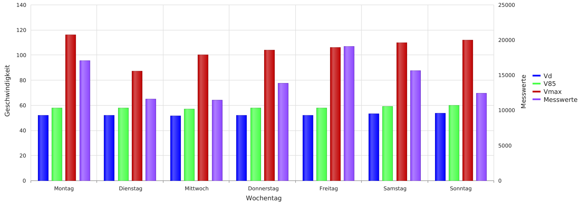
2024_12_13-2025_03_11 Norddrebber B214 Richtung Schwarmstedt Vd, V85, Vmax, Anzahl der Messwerte vs. Wochentag
