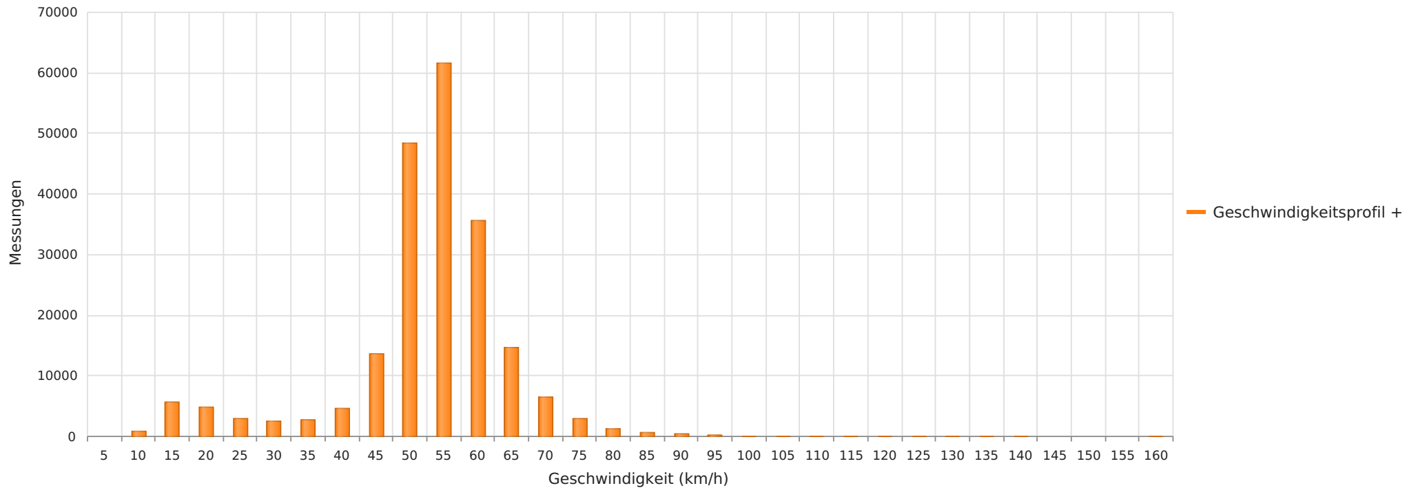
2024_12_13-2025_03_10 Marklendorf B214 Richtung Nienburg Anzahl der Messwerte vs. Geschwindigkeit
